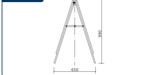
寸法図
