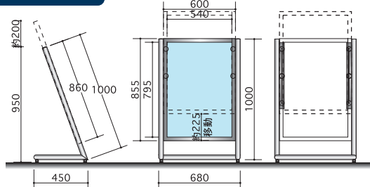
寸法図
